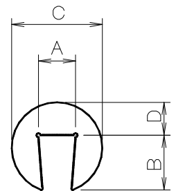
溝形ガード断面
